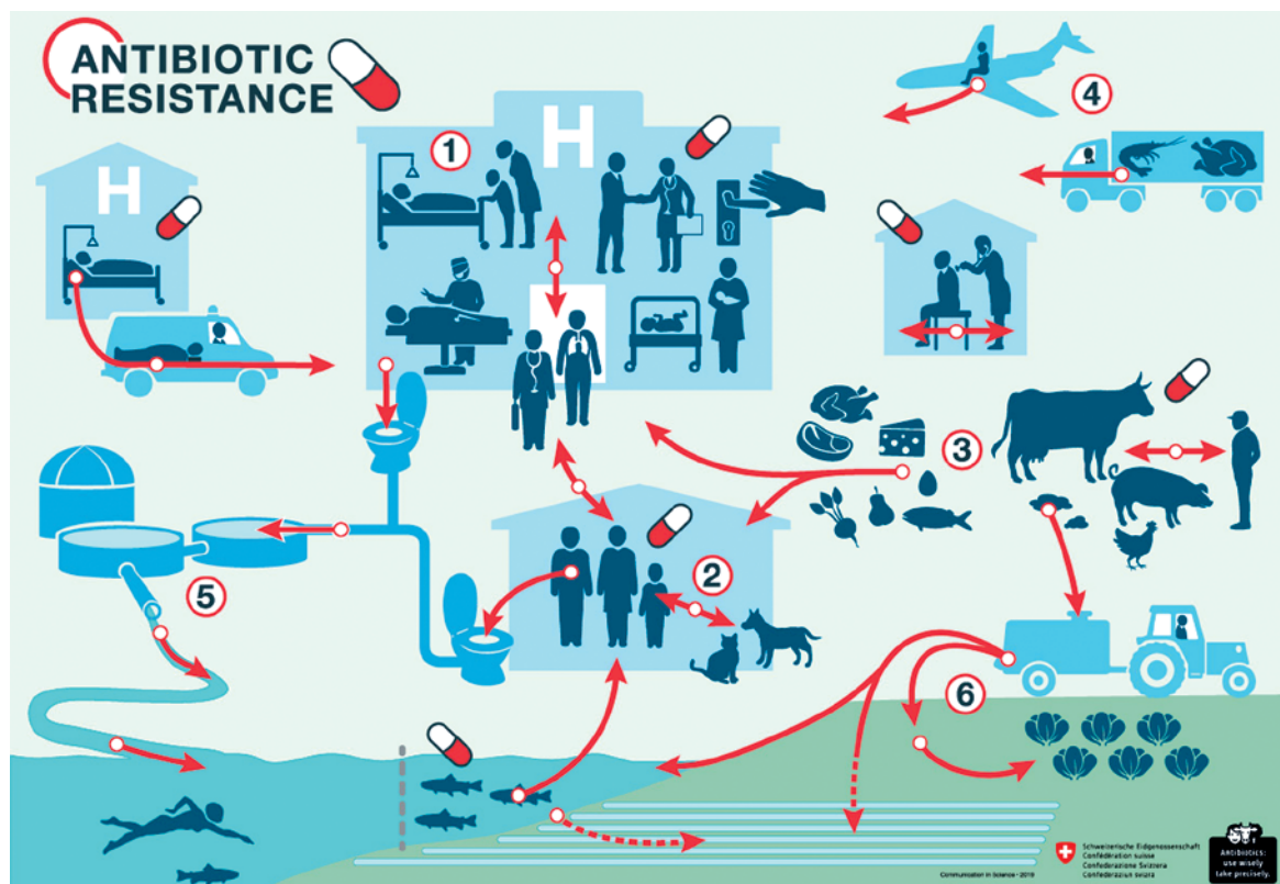
Abbildung 1: Ursachen und Übertragungswege von antibiotikaresistenten Bakterien [2].
